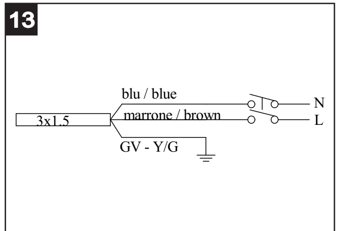
Schnittstellensignale (Abb.12)
